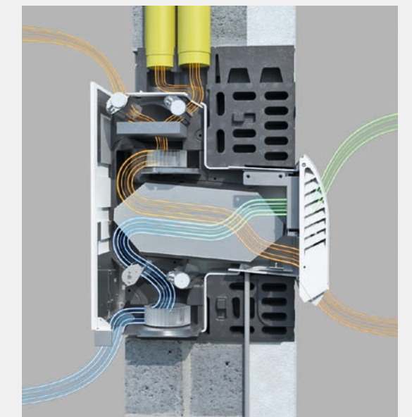
Querschnitt freeAir 100 mit Gegenstrom-Wärmetauscher
